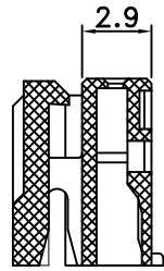
SECTION A-A ⑤
