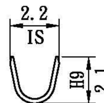
A-A Section
