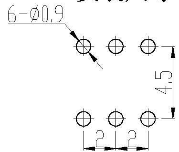
安装尺寸
